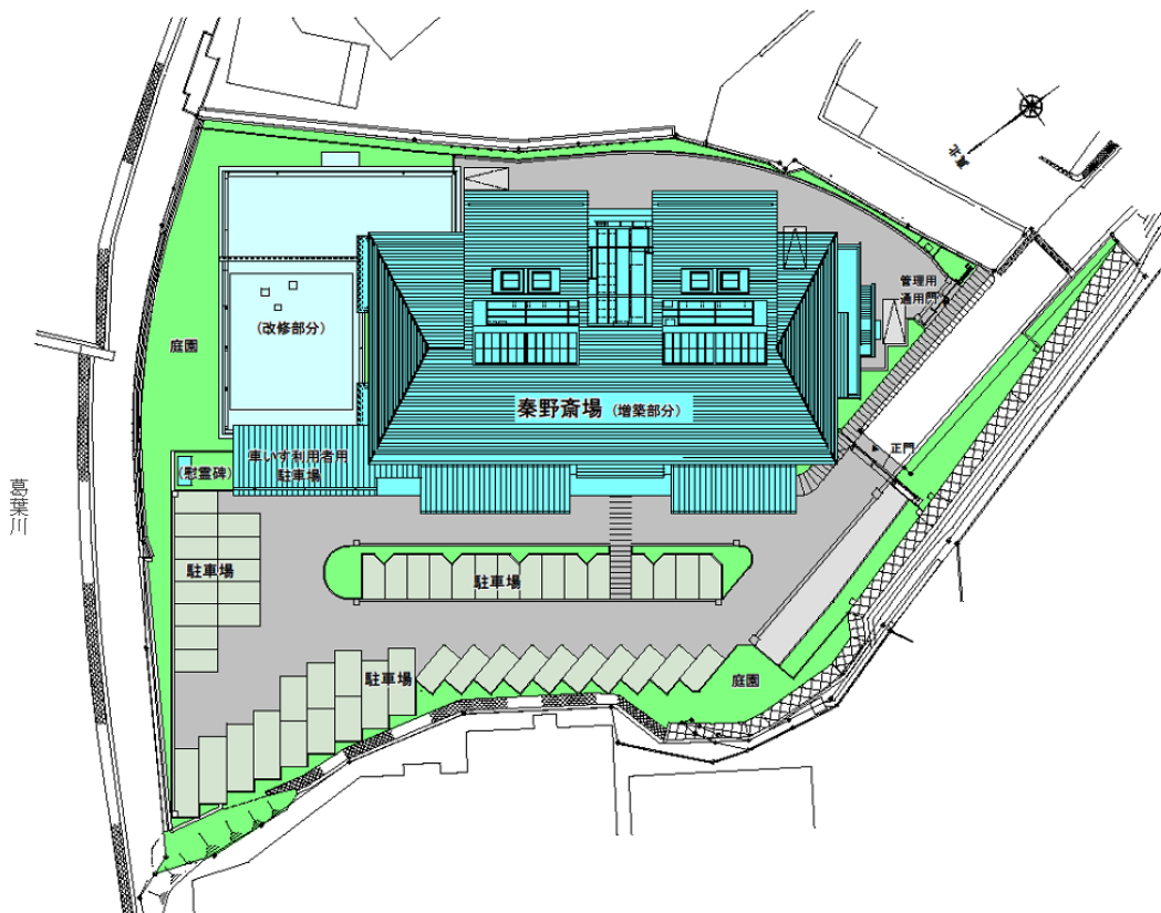
秦野斎場 施設配置図
