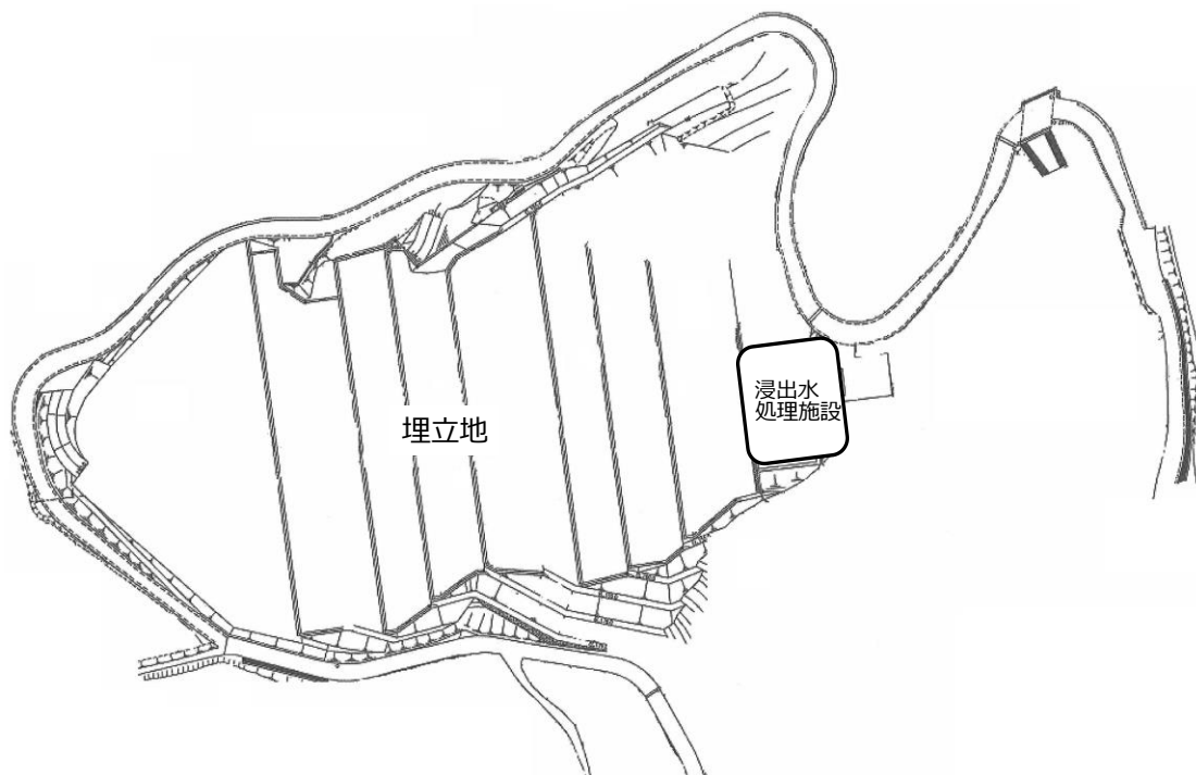
栗原一般廃棄物最終処分場 施設配置図
